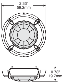
FSP-L2 dimensions
