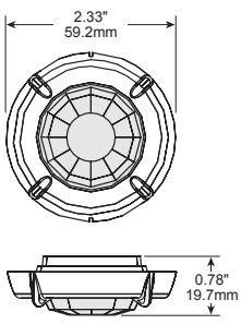
FSP-L2 dimensions
