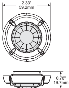
FSP-L2 dimensions
