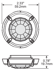
FSP-L2 dimensions
