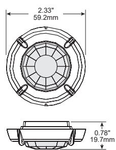
FSP-L2 dimensions
